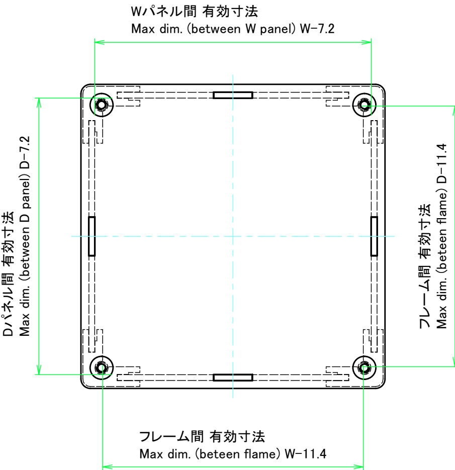
下カバー / Bottom cover
